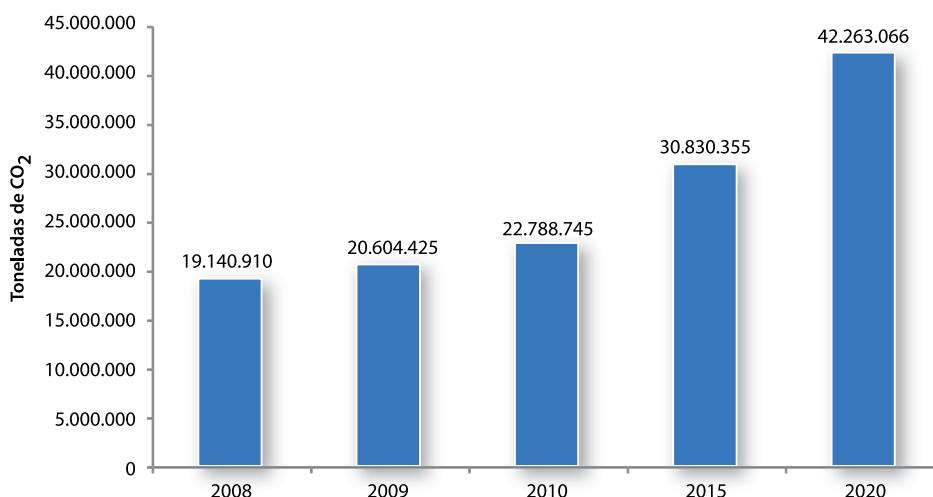
Gráfico 27. Emisiones de CO 2 evitadas en el período 2008-2010. Previsión 2015 y 2020
