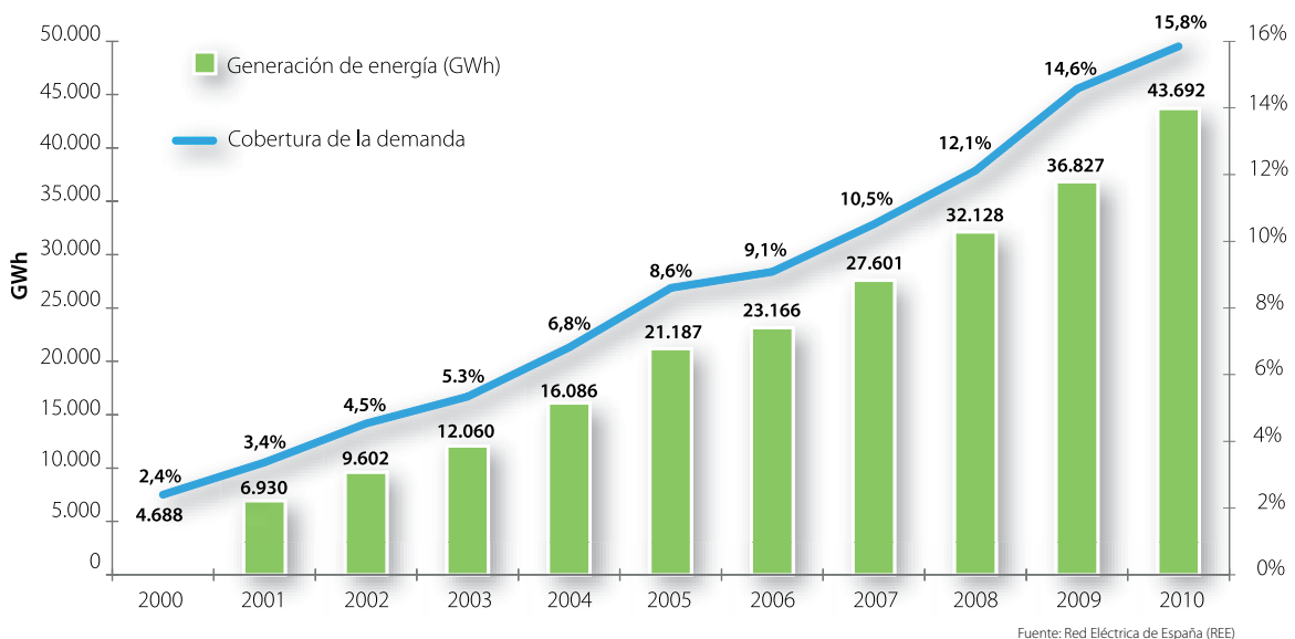
Gráfico 7. Generación de energía y porcentaje de cobertura de la demanda con eólica
